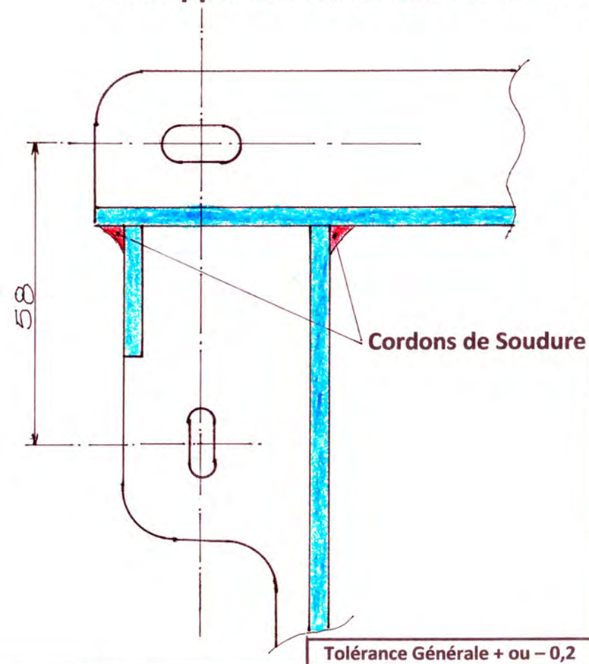
Schéma d'assemblage des Supports Bobines & Avertisseur
