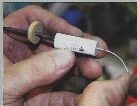
25 Recourber légèrement l'extrémité libre de la capacité.
