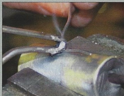
30 Un petit étamage pour "souder" le fil sur le corps.
