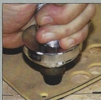
22 Il nous faut réaliser la rondelle caoutchouc d'étanchéité à l'emporte-pièce.
