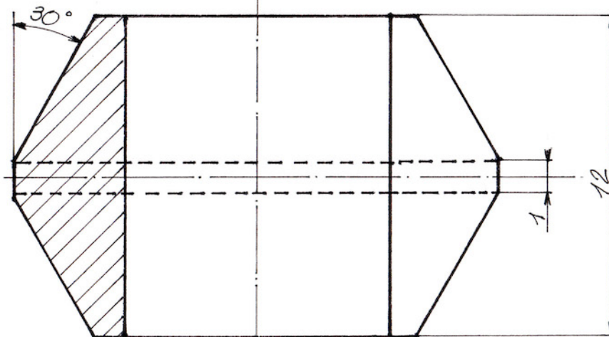
Coupe A-A
