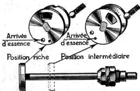
Fig. 27. — Tirette et glaces du bistarter.
