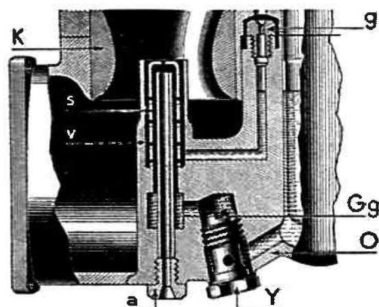
Fig. 30. — Montage 20 en coupe.
