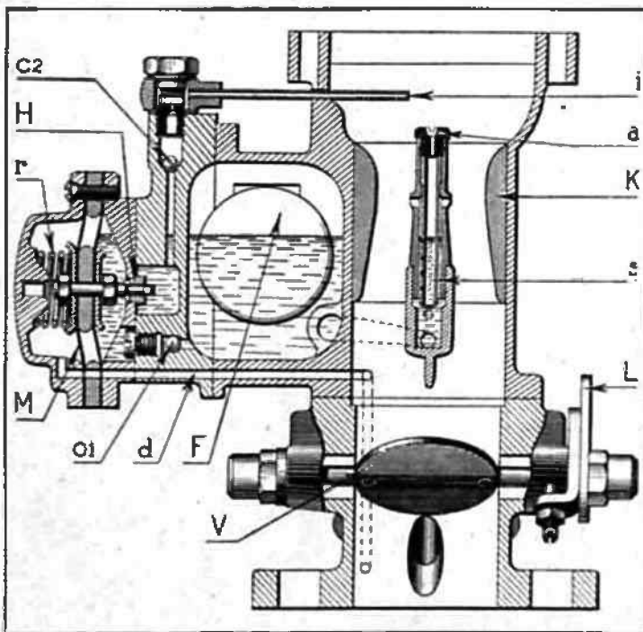
Fig. 18. — Coupe transversale du carburateur Inversé type 35 FAIP à bistarter, montage 21. Pompe à membrane.
