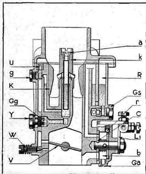
Fig. 12. — Coupe du Solex inversé 30 IA à bistarter, Montage 20.
