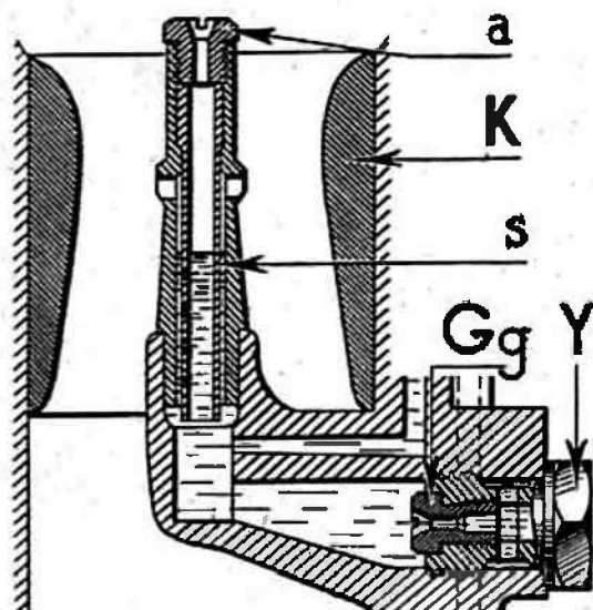
Fig. 31 — Montage 21 en coupe.
