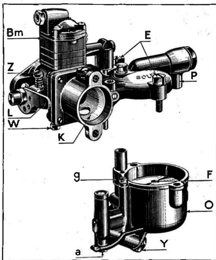
Fig. 2. — Solex horizontal type HTD à thermostarter. Montage 20. Ralenti à réglage d'essence
