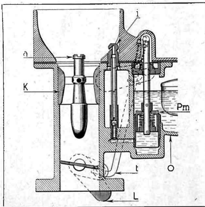
Fig. 22. — Coupe transversale du Solex double corps inversé type 30 FFIAP à bistarter. Pompe mécanique. Montage 21.
