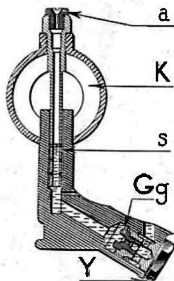
Fig. 32 — Montage 22 en coupe.
