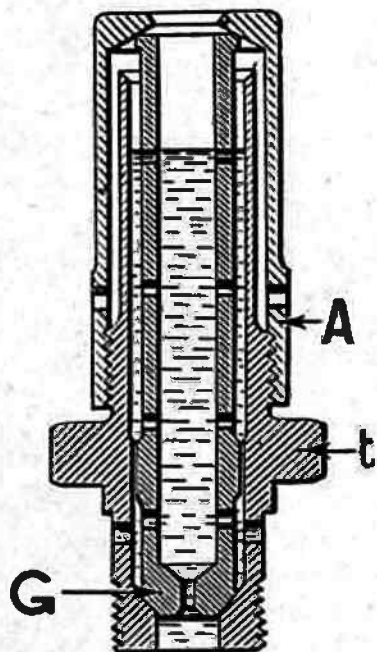
Fig. 29. — Montage 12 en coupe.
