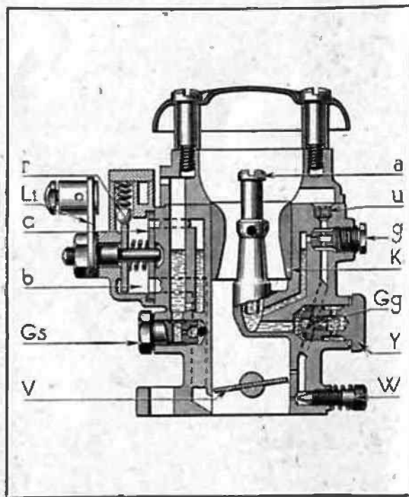
Fig. 11. — [Coupe longitudinale
