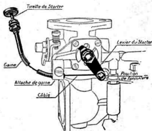
Fig. 25. — Montage de la tirette.
