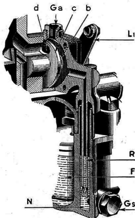
Fig. 26. — Le starter.
