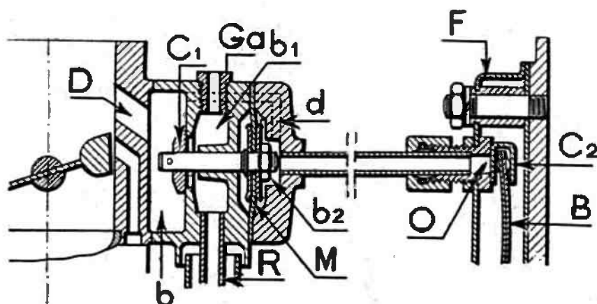
Fig. 28. — Coupe du thermostarter à membrane.
