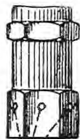
Fig. 18 CHAPEAU DE GICLEUR 13×300 (Carburateur FH)
