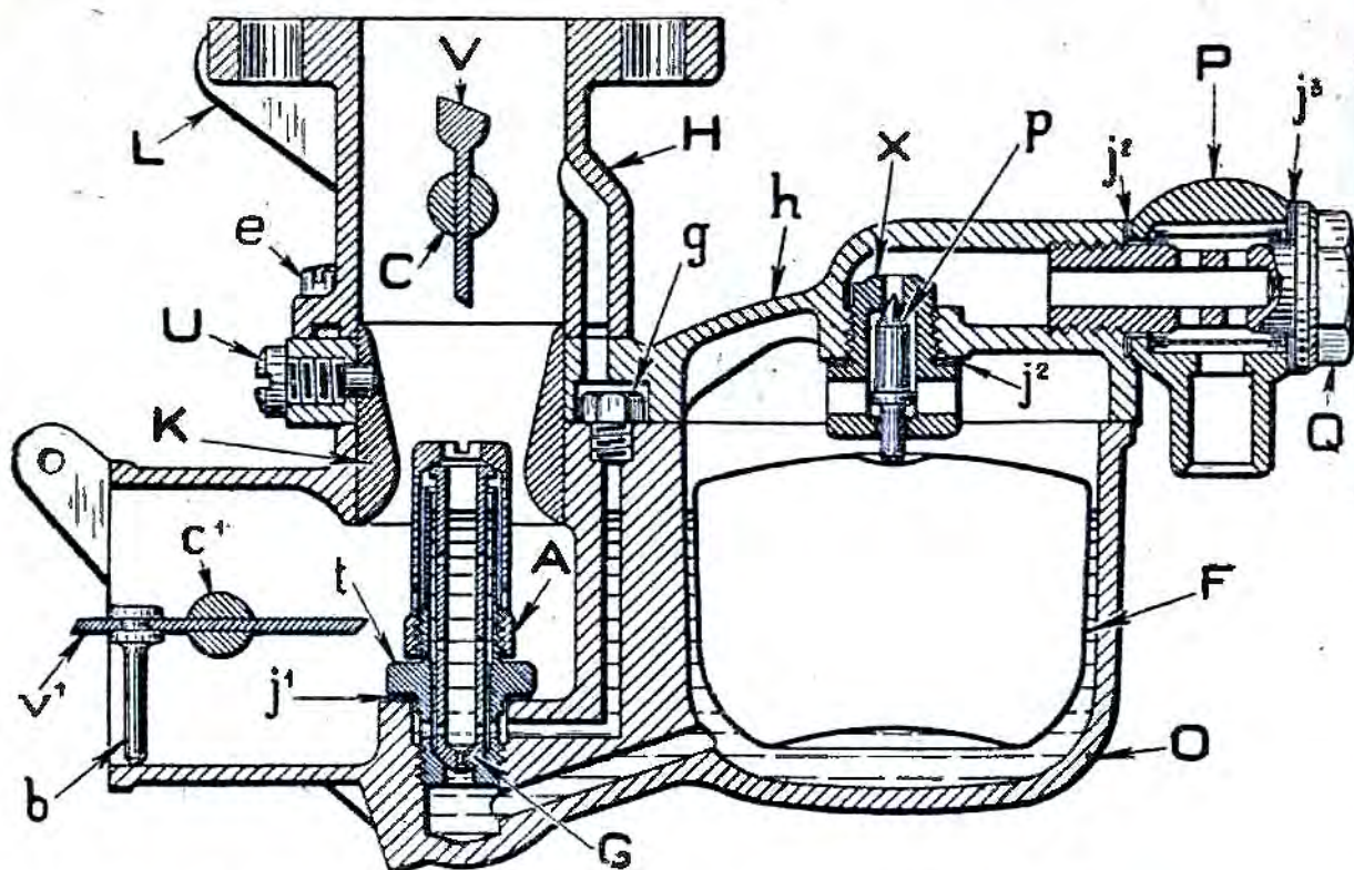
I Fig 3. — Coupe du carburateur vertical Type 26 FV
