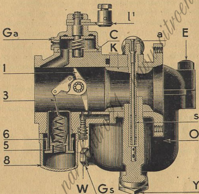
Fig. 2. — Carburateur-régulateur Solex horizontal
