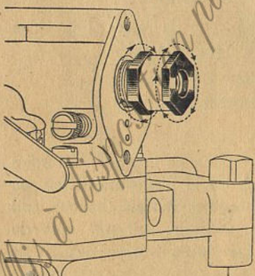
Fig. 5. — Pour donner de la stabilité et éviter le " pompage " du moteur
