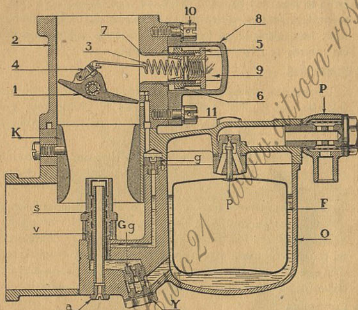
Fig. 1. — Coupe du carburateur-régulateur Solex vertical
