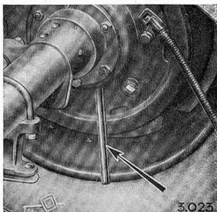
Fig. 21. — Tube d'évacuation d'huile des freins arrière.
