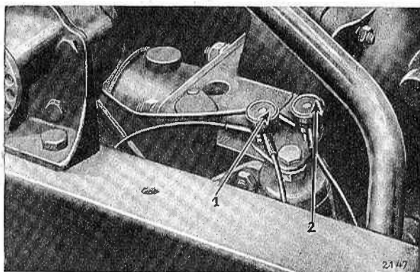
Fig. 55. — Fusibles de protection.
