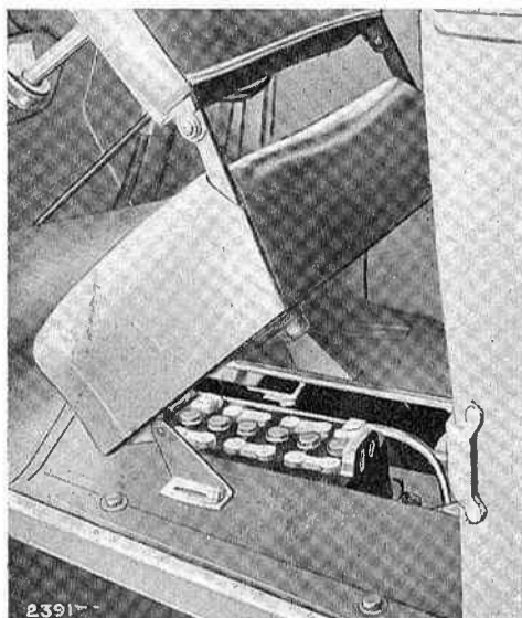
Fig. 28. — Accessibilité des accumulateurs. Les 2 bouchons de gauche sont facilement accessibles siège baissé, les 4 bouchons de droite peuvent être atteints siège levé comme indiqué sur la figure.
