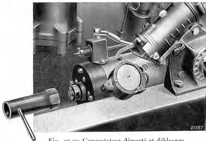
Fig. 27.— Commutateur démonté et déblocage du démarrreur (tourner la clé dans le sens des aiguilles d'une montre).
