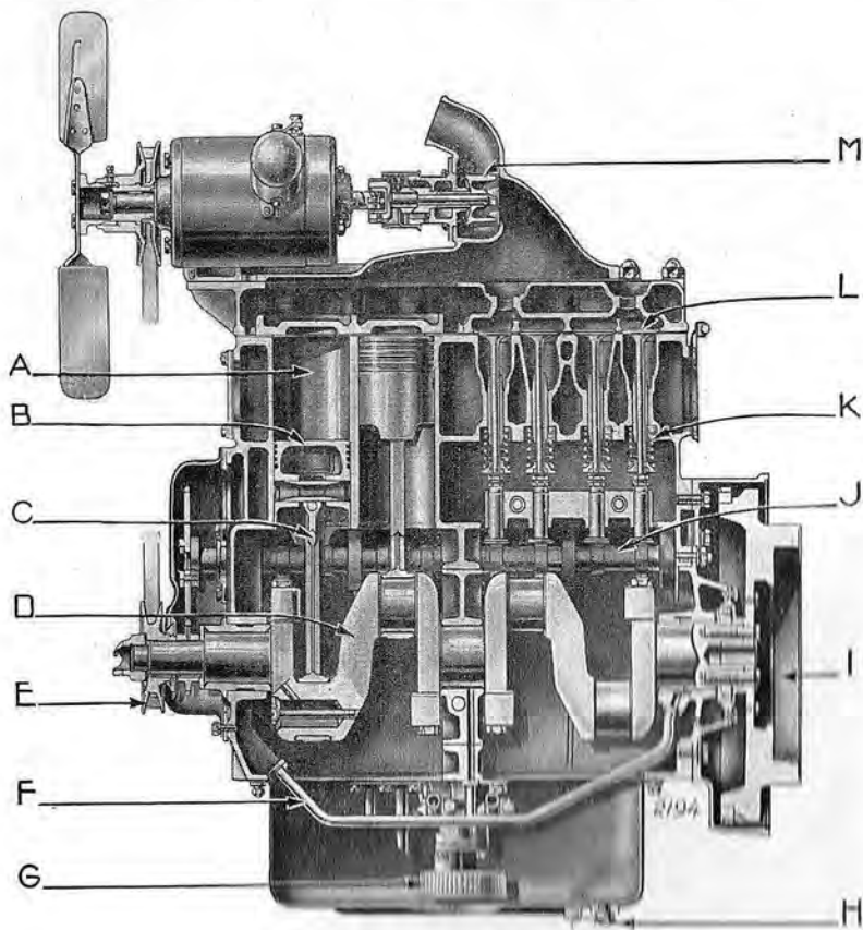
Fig. 4. — Coupe longitudinale du moteur.
