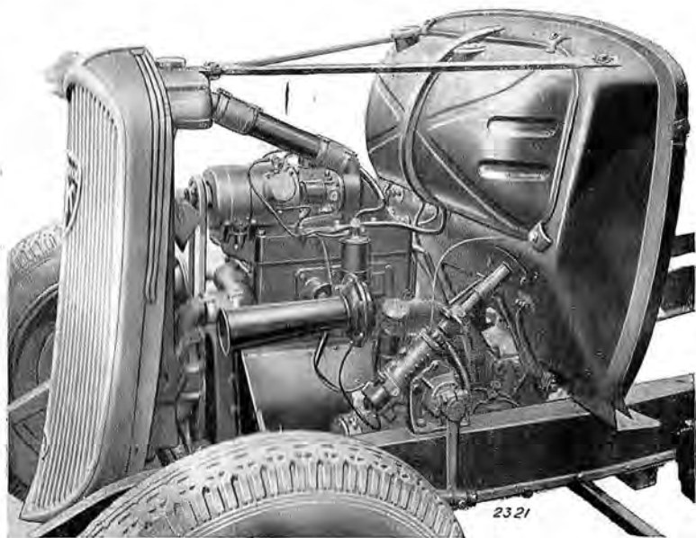
Fig. 21. — Vue du moteur côté gauche.
