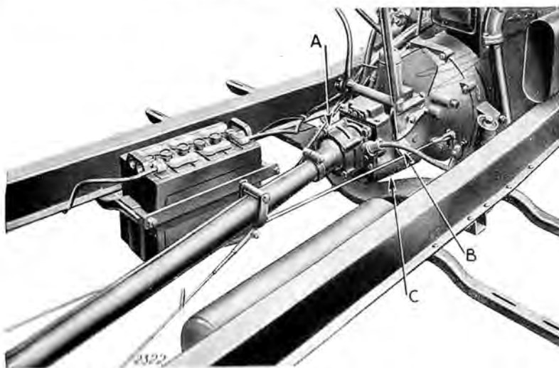
Fig. 22. — Vue de la boîte de vitesses et du joint de cardan.
