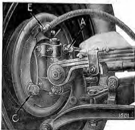
Fig. 16. — Réglage des freins avant.
