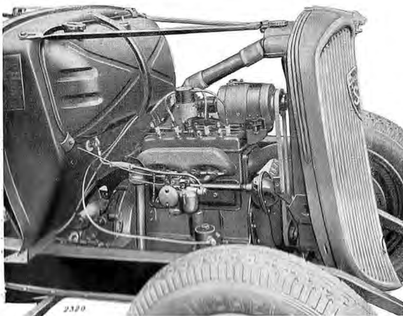
Fig. 20. — Vue latérale droite du moteur montrant nettement la commande du régulateur.
