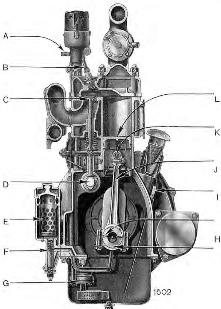
Fig. 5. — Coupe transversale du moteur.
