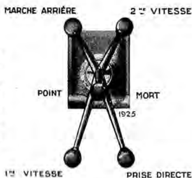
Fig. 29. — Schéma des positions du levier des vitesses des boîtes "standard" synchronisées.
