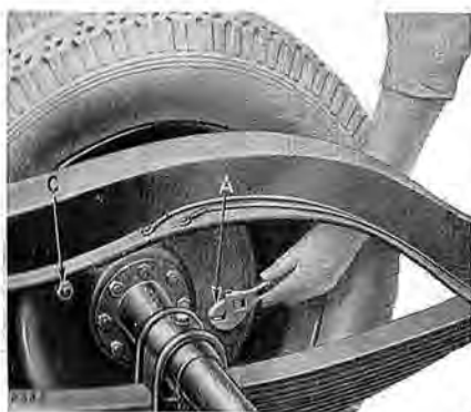
Fig. 17. — Réglage des freins arrière.
