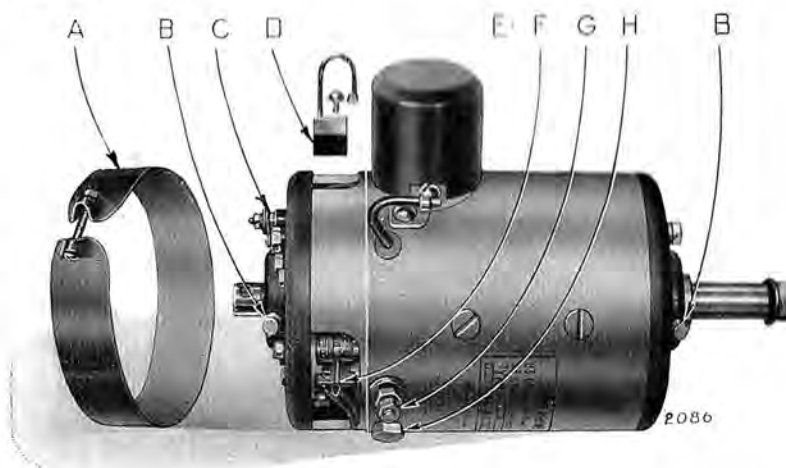
Fig. 26. — Vue de la dynamo avec sangle enlevée (nouvelle dynamo compound)
