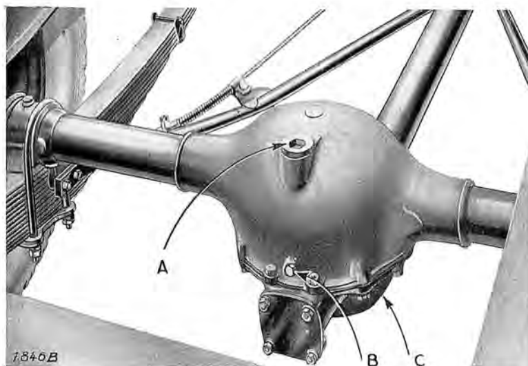
Fig. 23. — Graissage du pont arrière : A) Bouchon de remplissage ; B) Bouchon de niveau ; C) Bouchon de vidange.
