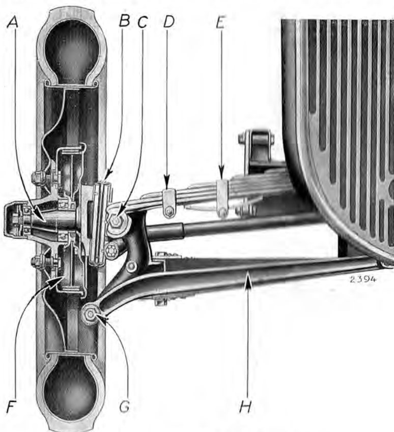
Fig. 9. — Coupe de l'essieu avant droit.
