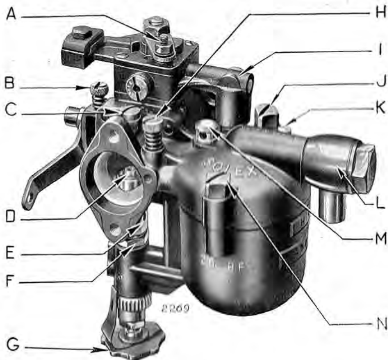
Fig. 11. — Carburateur.
