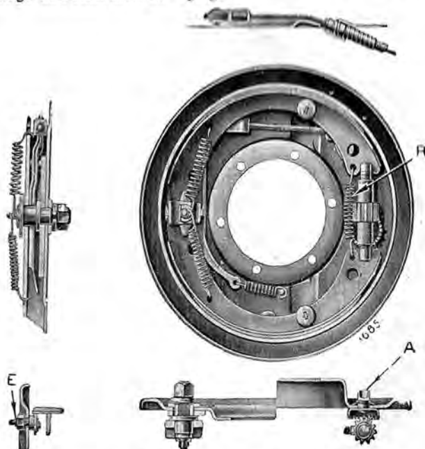
Fig. 18. — Vue intérieure et détails d'un tambour de frein.
