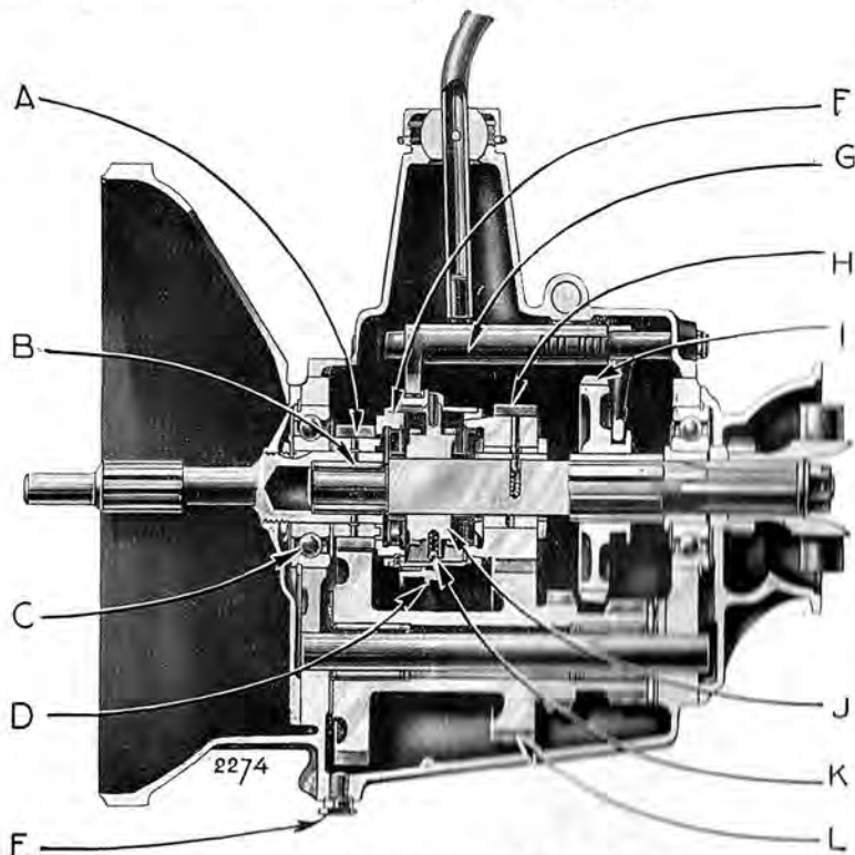
Fig. 7. — Coupe longitudinale de la boîte de vitesses.
