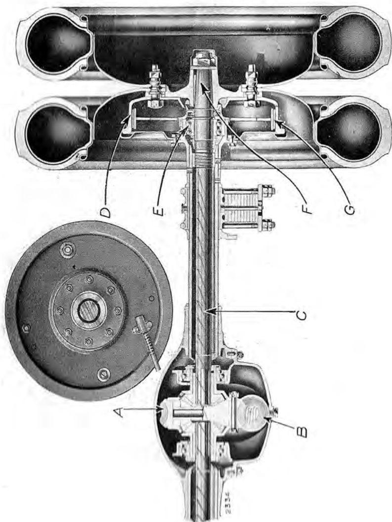
Fig. 15. — Coupe du pont arrière et vue d'un frein.
