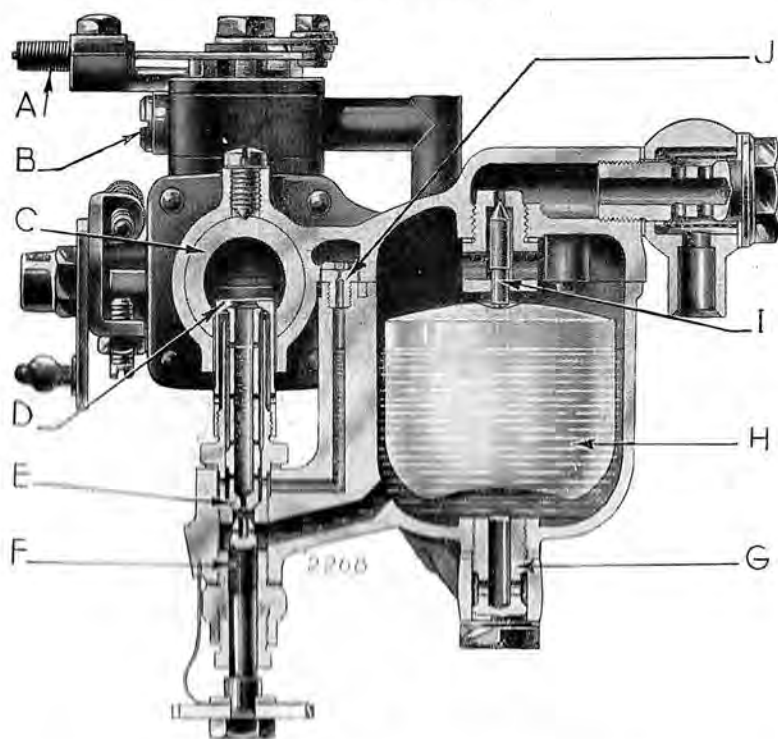
Fig. 10. — Fausse coupe montrant le fonctionnement du dispositif starter pour départ à froid.
