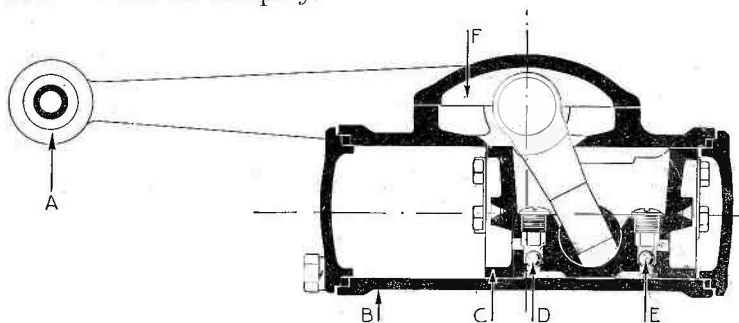
Fig. 12. — Coupe longitudinale.
