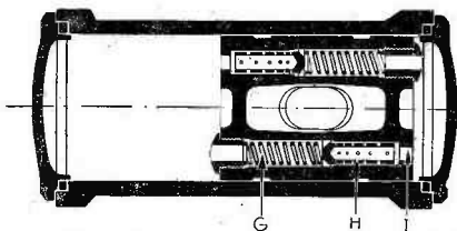
Fig. 13. — Coupe schématique montrant le fonctionnement des amortisseurs.
