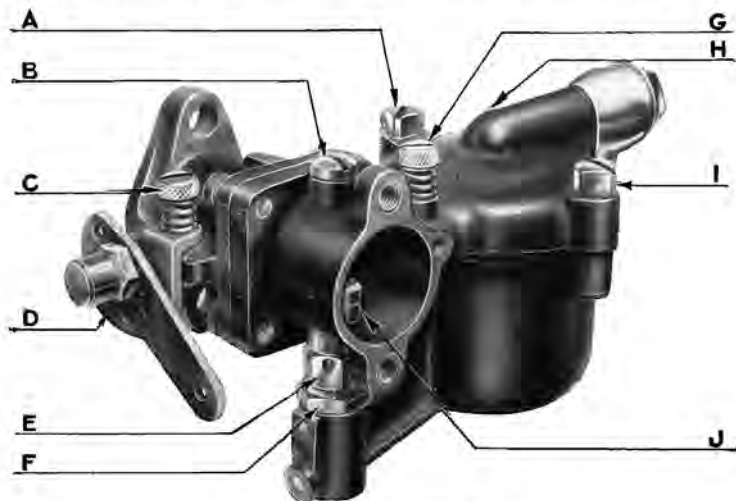
Fig. 9. — Carburateur.
