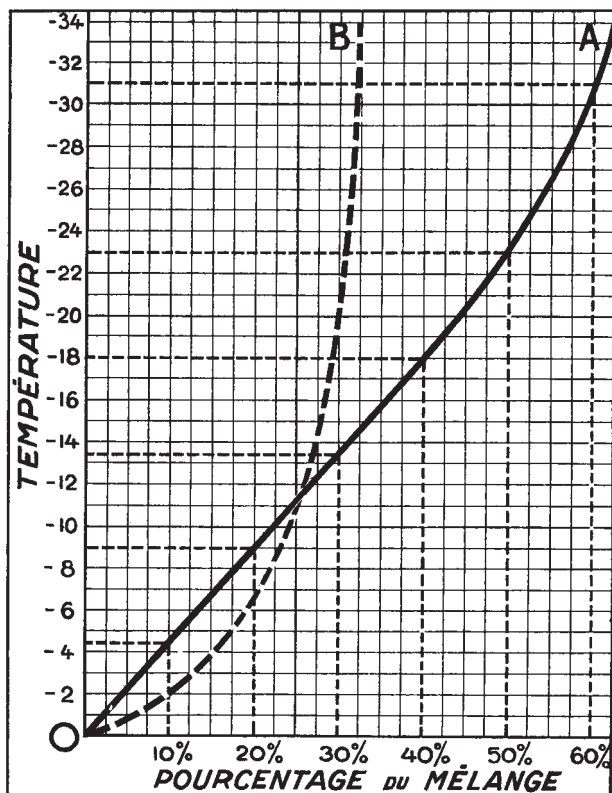
Fig. 27. — Pourcentage pour les mélanges antigel.
