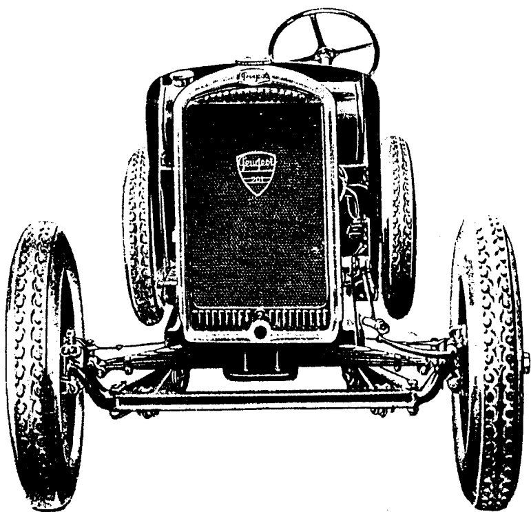
Fig. 1. — Vue de face du châssis.
