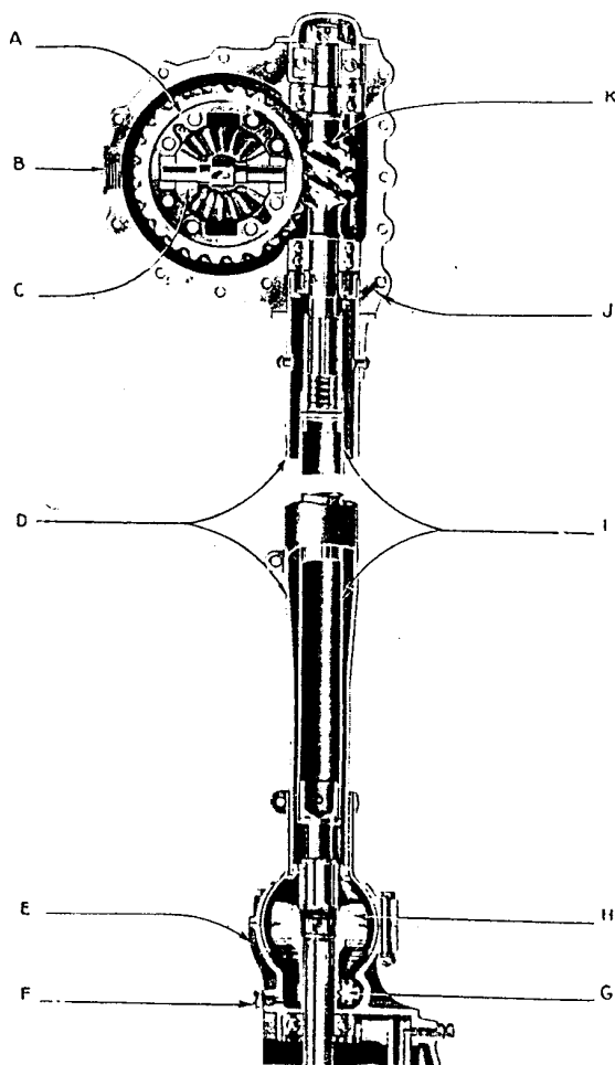
Fig. 8. — Coupe de l'arbre de transmission.
