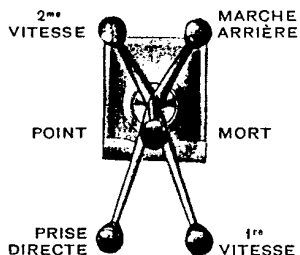
Fig. 24. — Schéma des positions du levier des vitesses.
