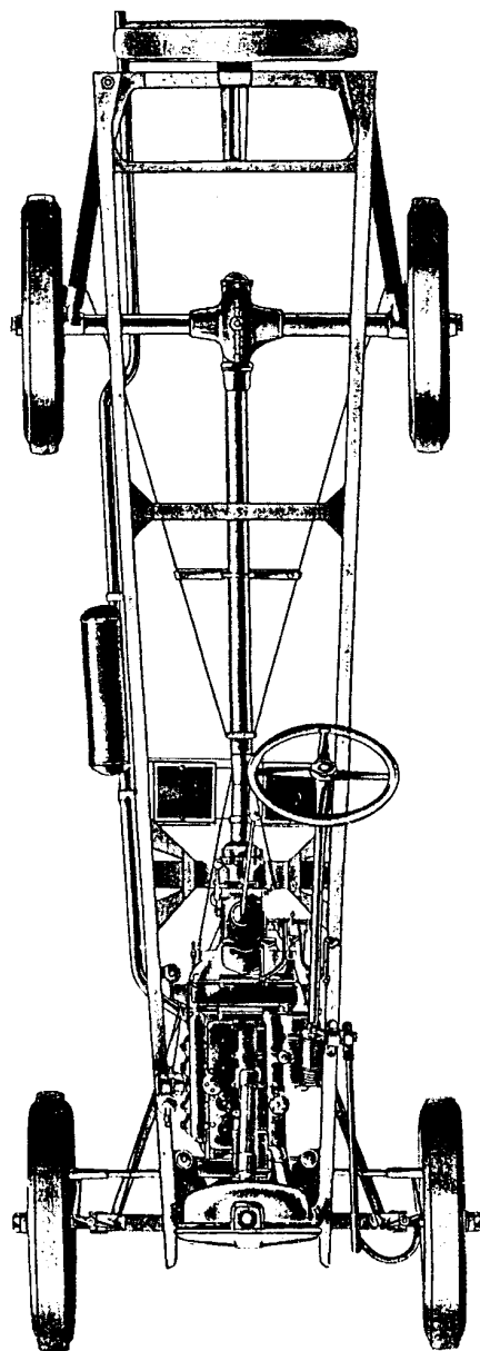
Fig. 3. — Vue en plan du châssis.
