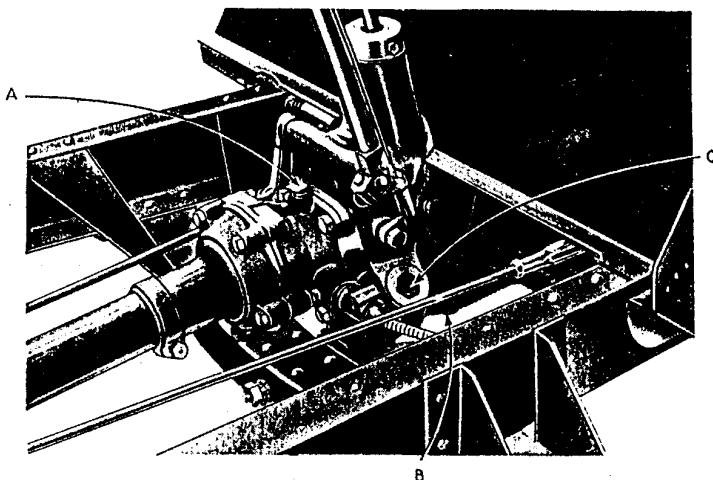
Fig. 17. — Graissage de la boîte de vitesses et du joint de cardan.
