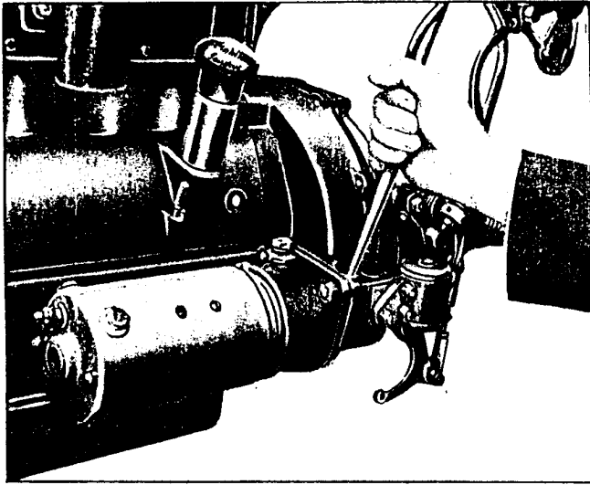
Fig. 20. — Déblocage du pignon de démarreur.
