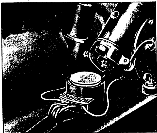
Fig. 22. — Commutateur démonté.
