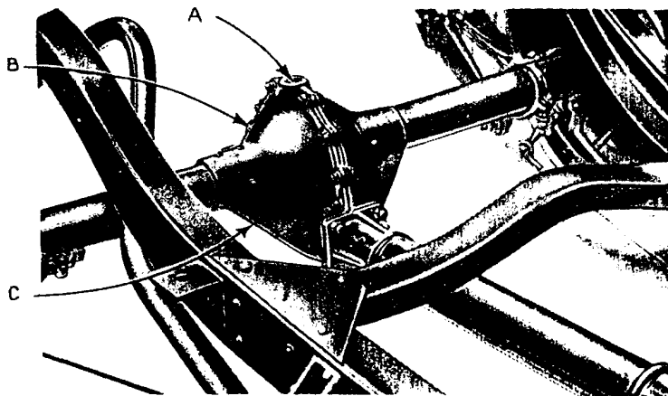
Fig. 18. — Graissage du pont arrière : A) Bouchon de remplissage ; B) Bouchon de niveau ; C) Bouchon de vidange.
