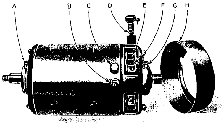
Fig. 19. — Dynamo.
