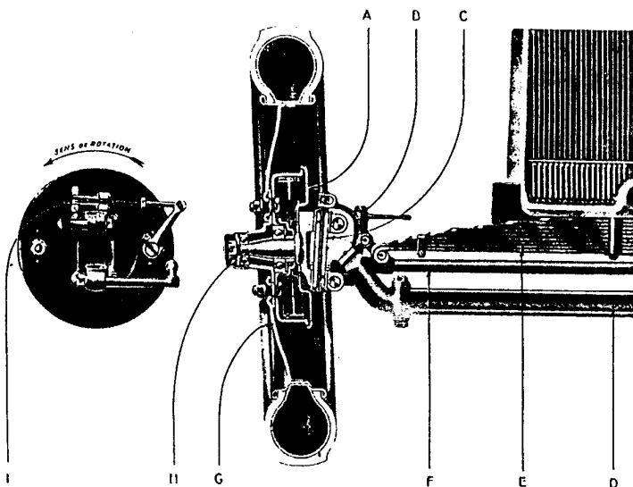
Fig. 6. — Coupe de l'essieu avant.
