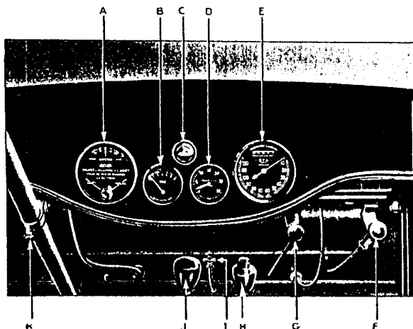
Fig. 23. — Groupement des organes de manœuvre et de contrôle.
