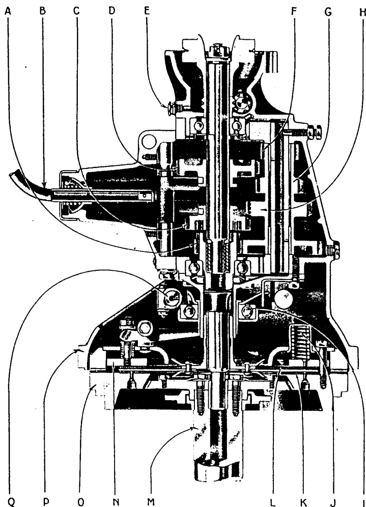
Fig. 11. — Embrayage et boîte de vitesses.
