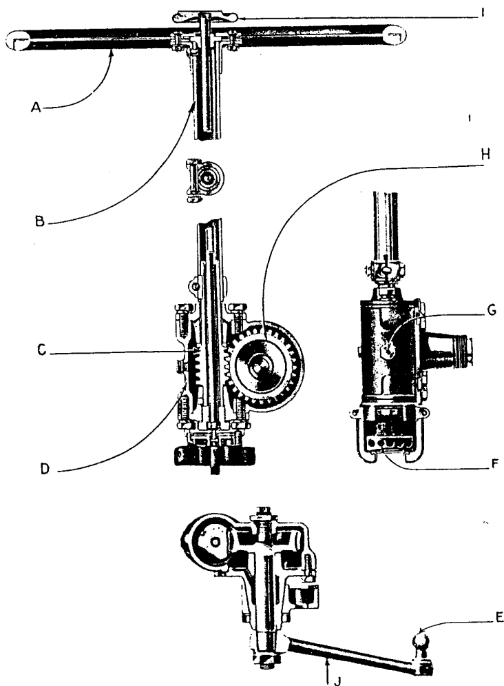
Fig. 12. — Coupe de la direction.
