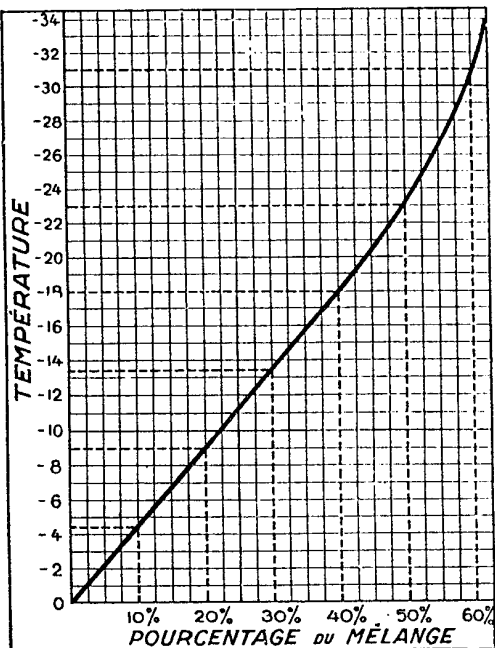
Fig. 25. — Pourcentage des mélanges alcool et eau pour éviter la congélation.
