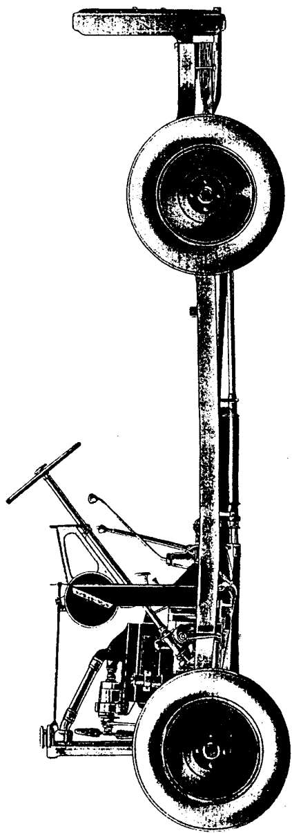
Fig. 2. — Vue latérale du châssis.
