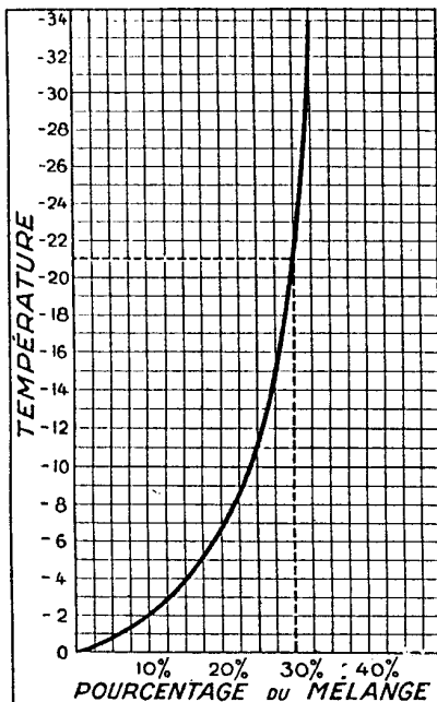
Fig. 26. — Pourcentage du mélange eau, alcool, glycérine, pour éviter la congélation
