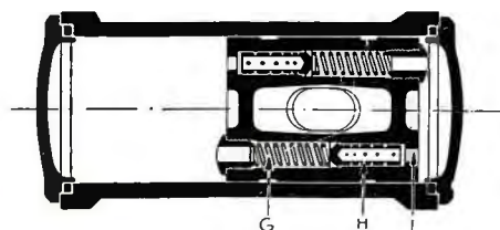
Fig. 12. — Coupe schématique montrant le fonctionnement des amortisseurs.
