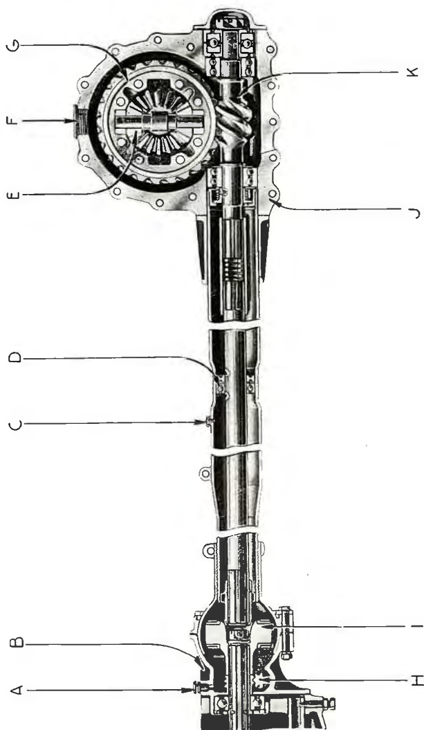
Fig. 8. — Coupe de l'arbre de transmission.
