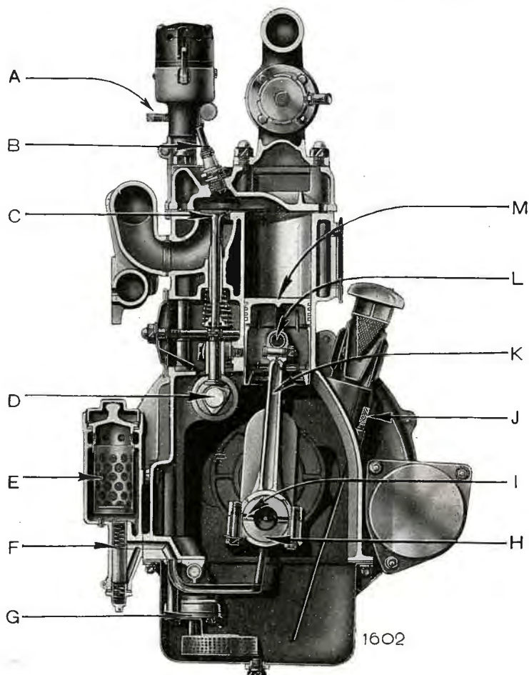
Fig. 5. — Coupe transversale du moteur.
