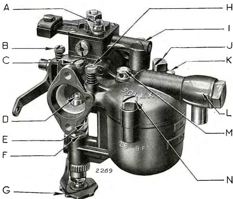
Fig. 15. — Carburateur.
