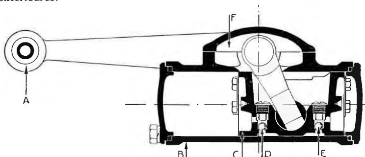
Fig. 11. — Coupe longitudinale.
