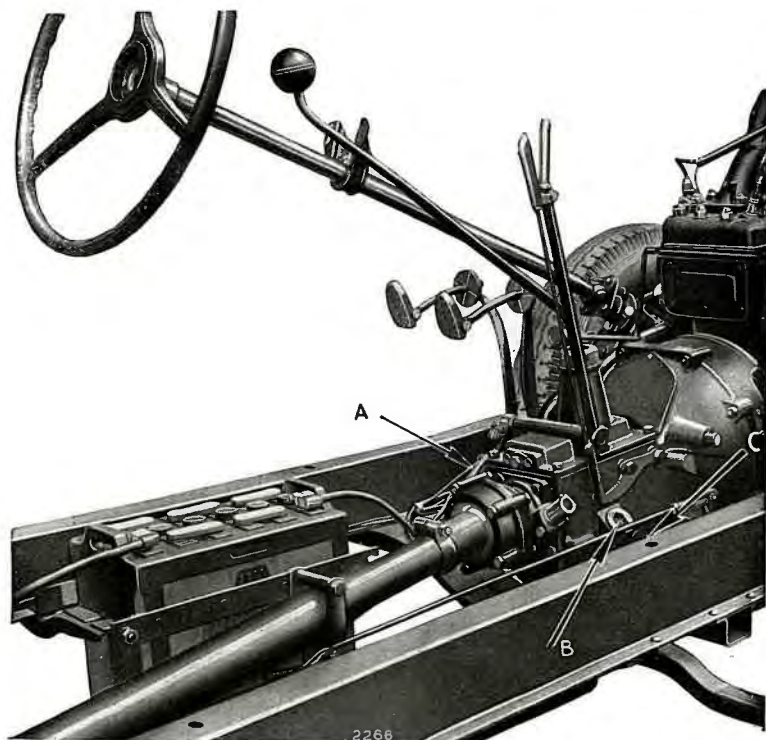
Fig. 25. — Vue de la boîte de vitesses et du joint de cardan.
