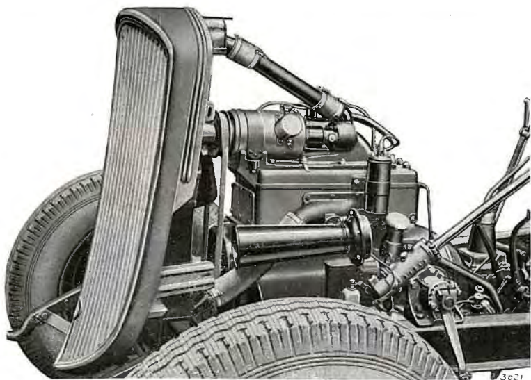
Fig. 25. — Vue latérale gauche du moteur.
