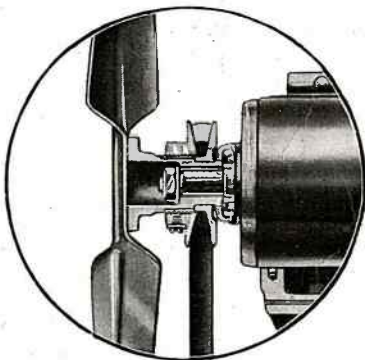
Fig. 18. — Ventilateur.
