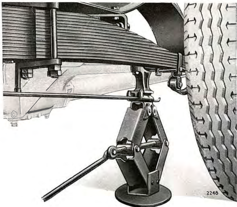
Fig. 15. — Montage du cric spécial.
