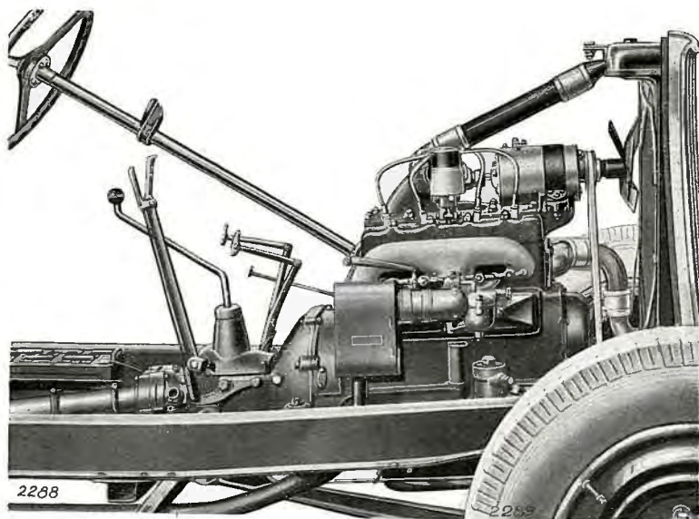
Fig. 16. — Vue latérale droite du moteur
