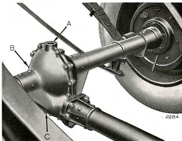
Fig. 26. — Graissage du pont arrière : A) Bouchon de remplissage ; B) Bouchon de niveau ; C) Bouchon de vidange.
