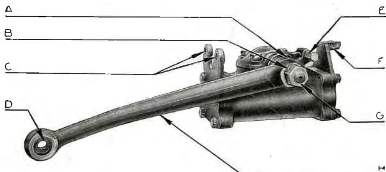
Fig. 10. — Amortisseur hydraulique.
