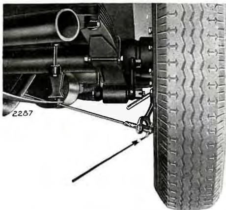
Fig. 21. — Réglage des freins arrière.
