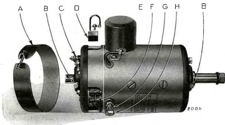
Fig. 29. — Vue de la dynamo avec sangle enlevée (nouvelle dynamo compound).
