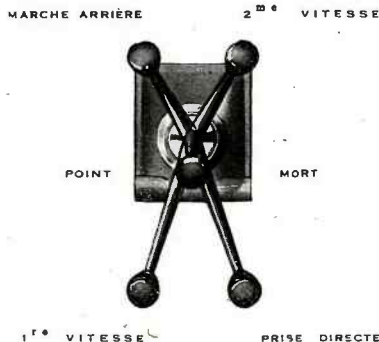
Fig. 32. — Schéma des positions du levier des vitesses des boîtes "standard" synchronisées.
