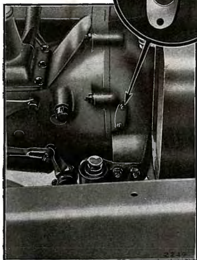
Fig. 17. Réglage de l'allumage.
