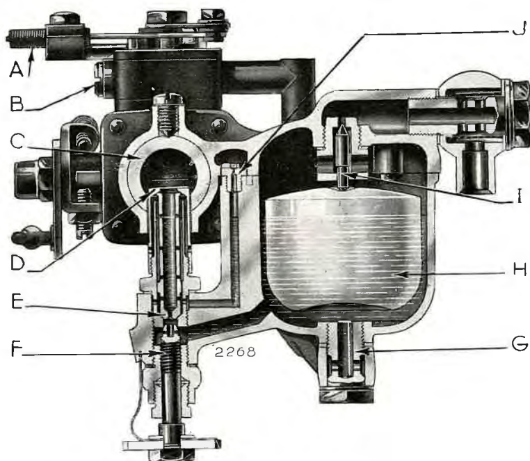
Fig. 14. — Coupe montrant les organes intérieurs du carburateur, notamment le dispositif appauvrisseur.
