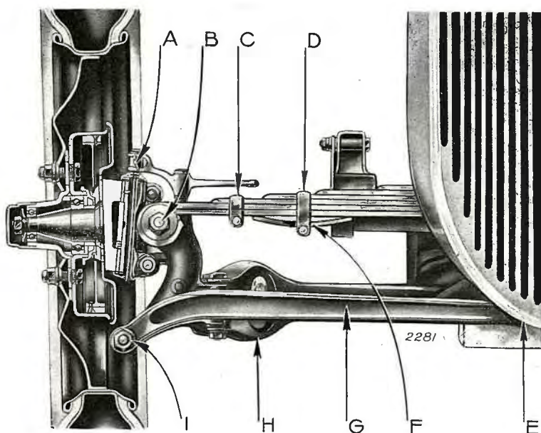
Fig. 9. — Coupe de l'essieu avant droit.
