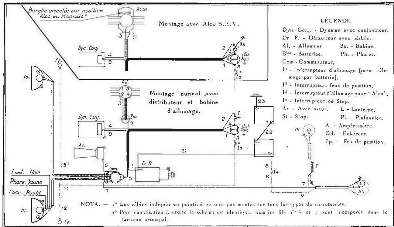
Fig. 52. — Schéma de l'installation électrique
