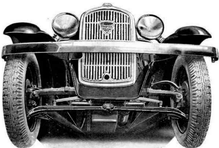
Fig. 1. — Vue du train AV. Peugeot à roues indépendantes type 301 C.
