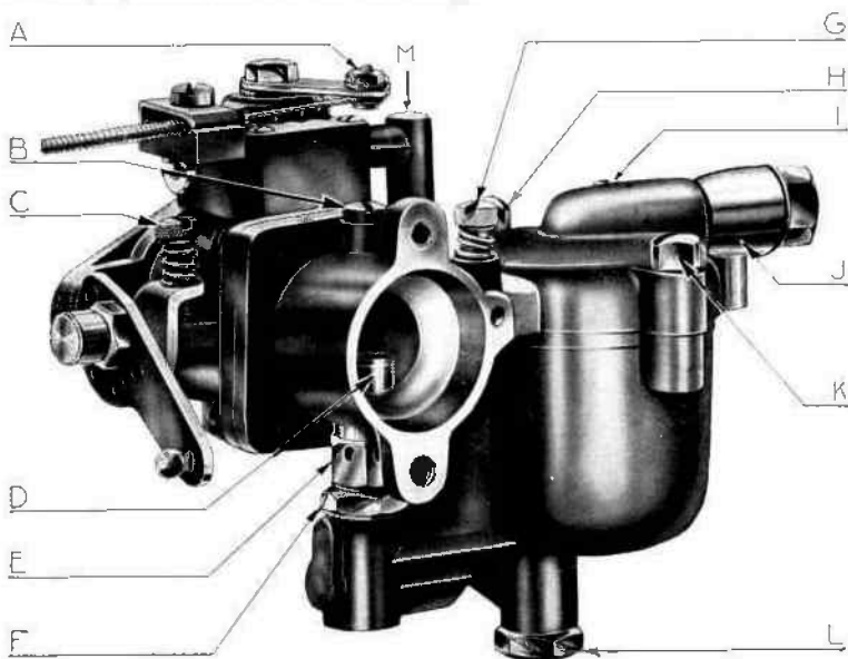
Fig. 17. — Carburateur.
