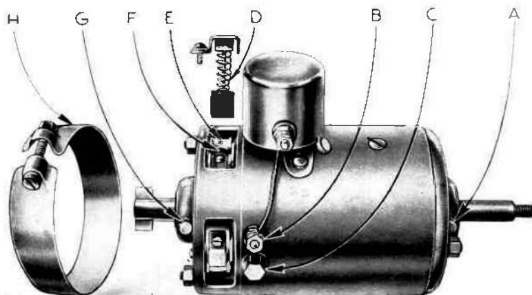
Fig. 30. — Dynamo.
