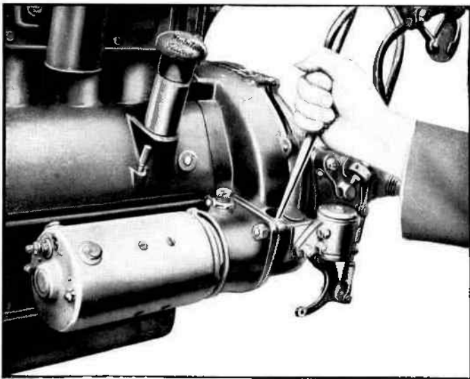
Fig. 31. — Déblocage du pignon de démarrage.
