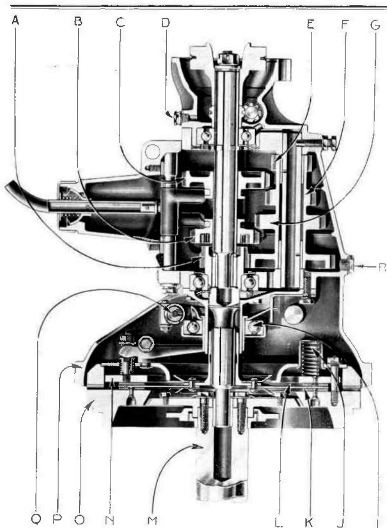
Fig. 20. — Embrayage et boîte de vitesses.
