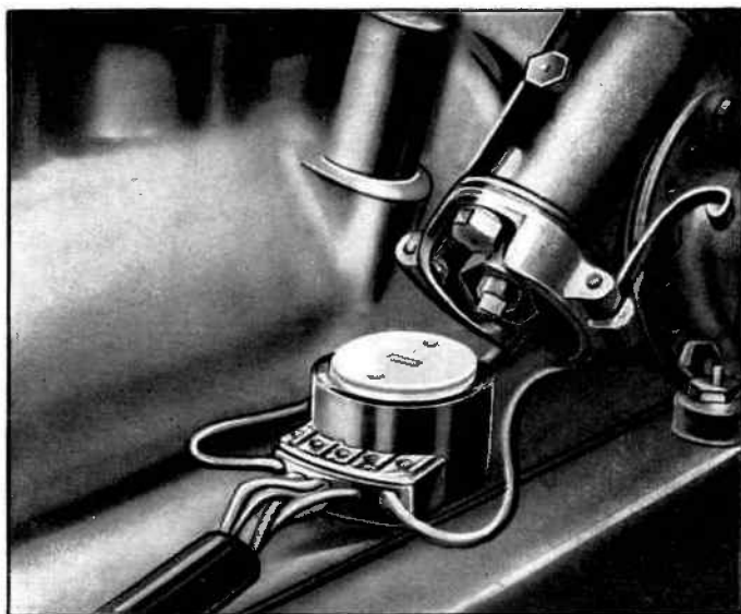
Fig. 33. — Commutateur démonté.
