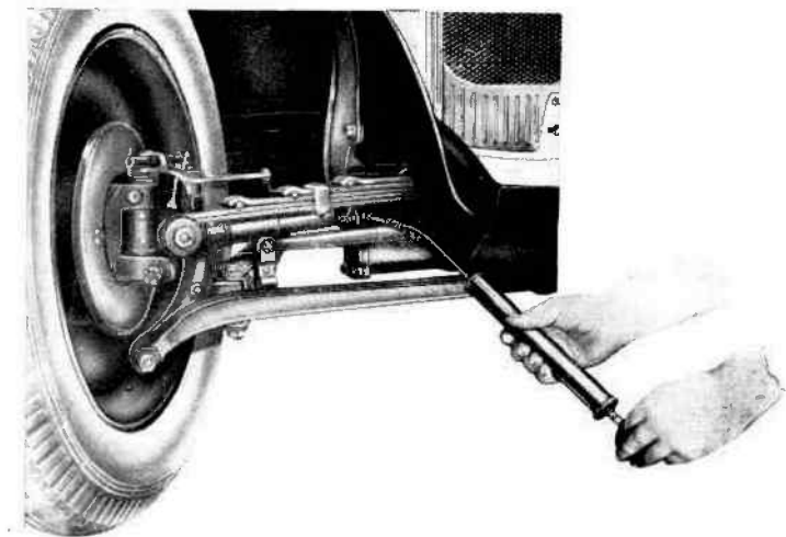
Fig. 14. — Remplissage à la seringue des amortisseurs.
