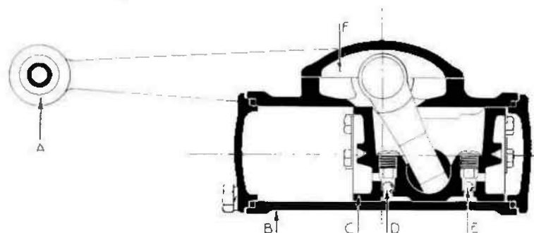
Fig. 11. — Coupe longitudinale.
