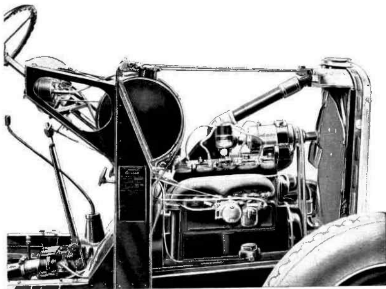
Fig. 3. — Vue avant droite du châssis.
