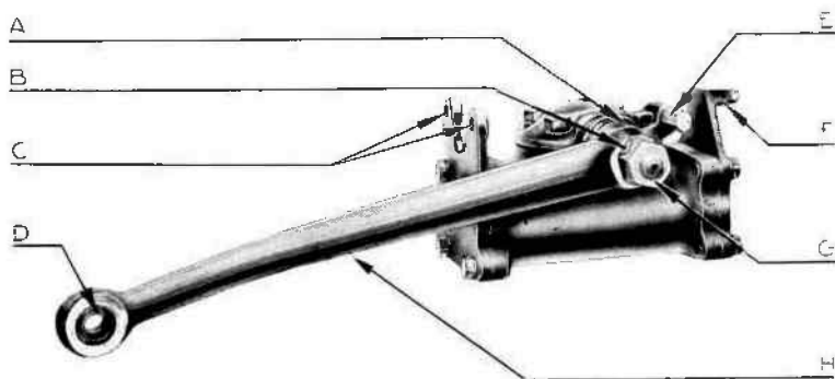
Fig 10. — Amortisseur hydraulique.
