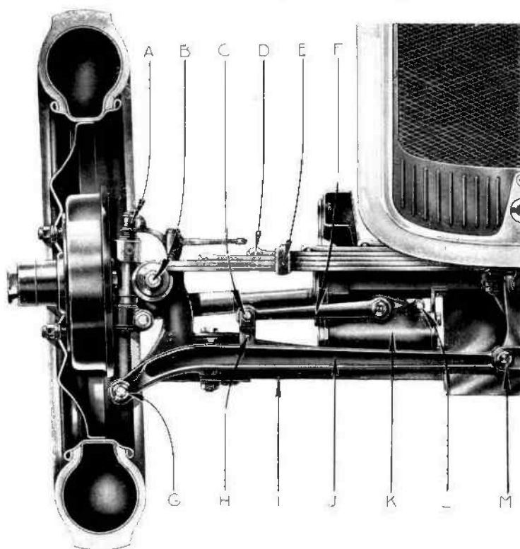
Fig. 9. — Coupe de l'essieu avant droit.
