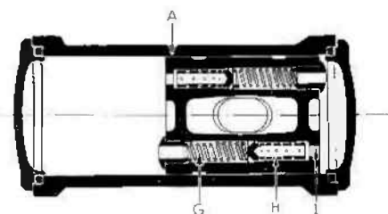
Fig. 12. — Coupe schématique montrant le fonctionnement des amortisseurs.
