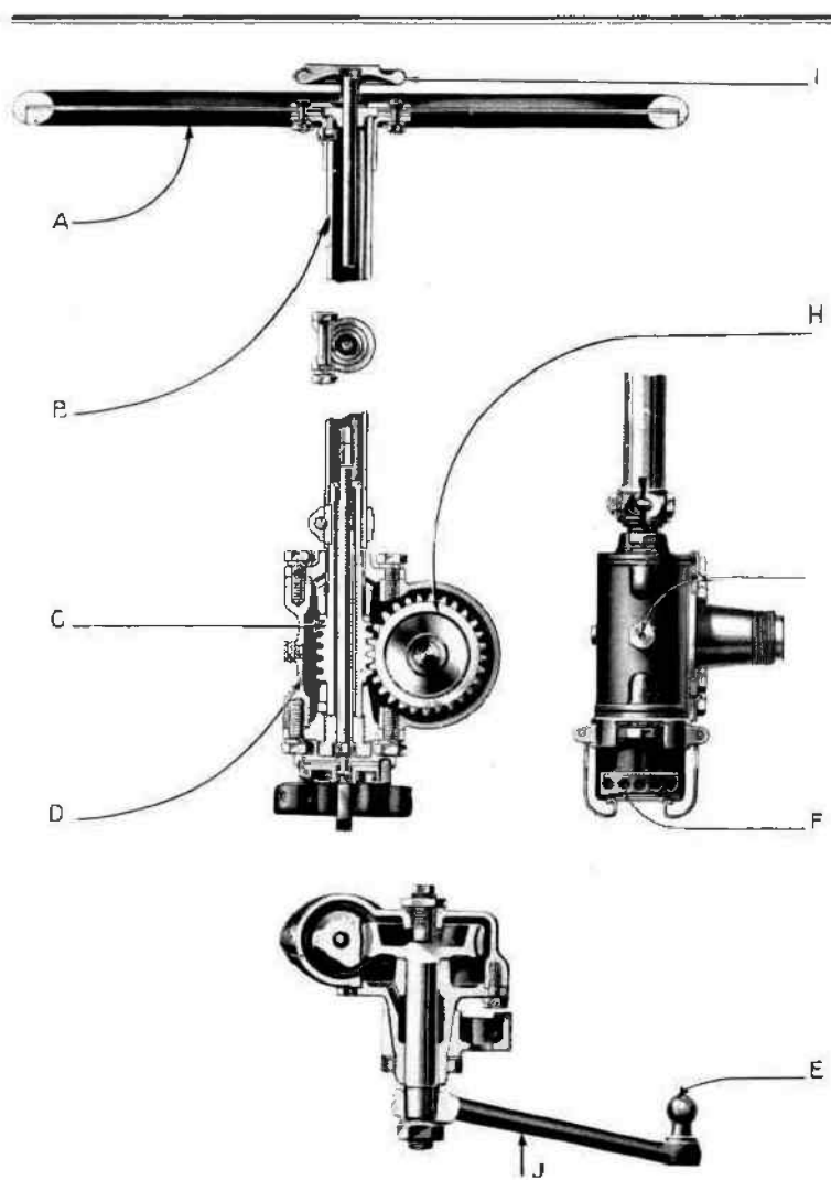
Fig. 21. — Coupe de la direction
