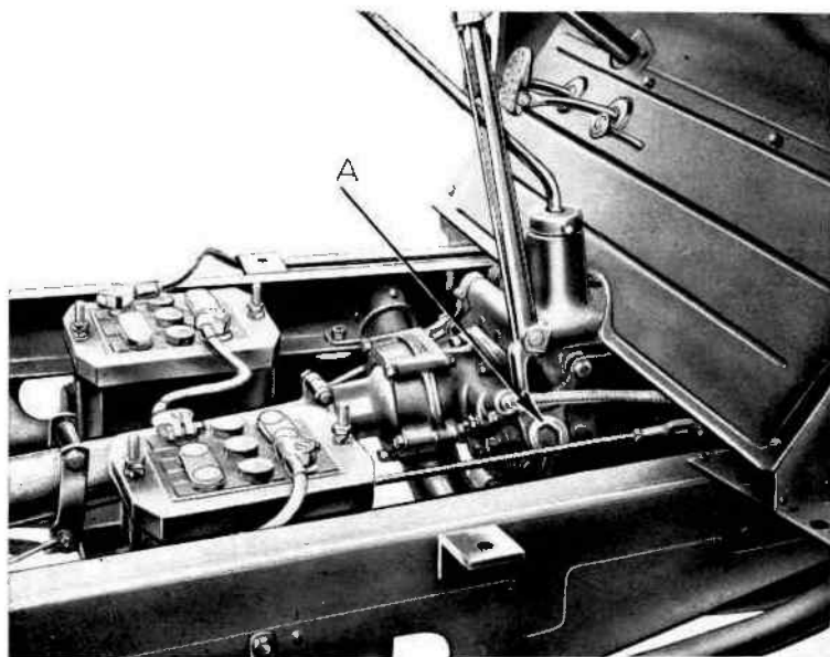
Fig. 26 — Graissage de la boîte de vitesses et du joint de cardan.
