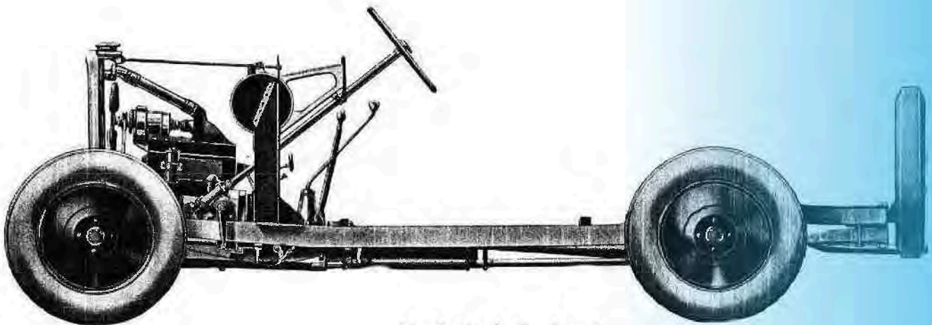
Vue latérale du châssis
