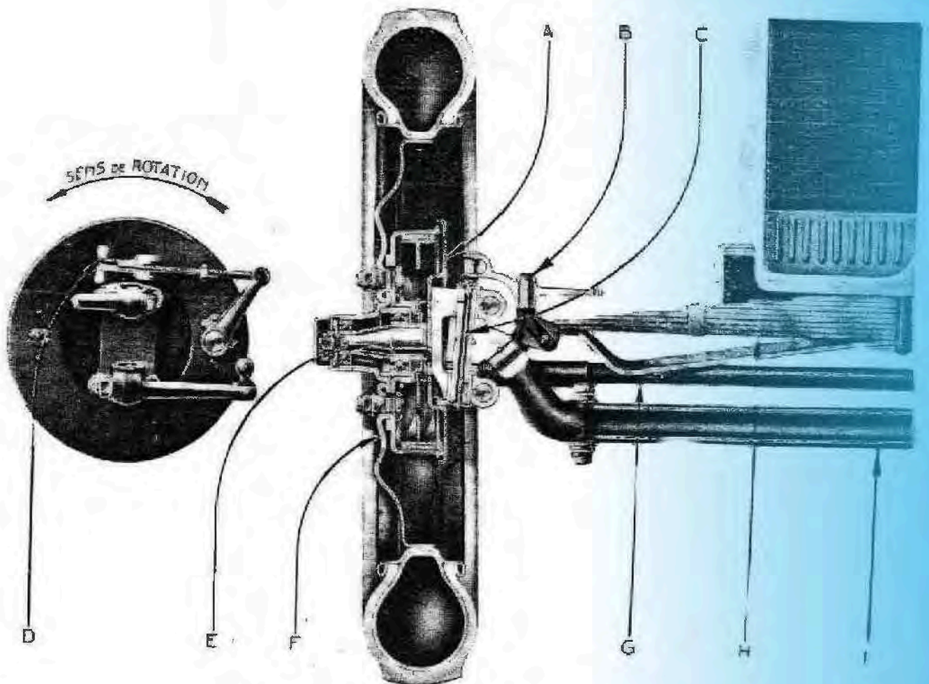
Fig. 6. — Coupe de l'essieu avant.
