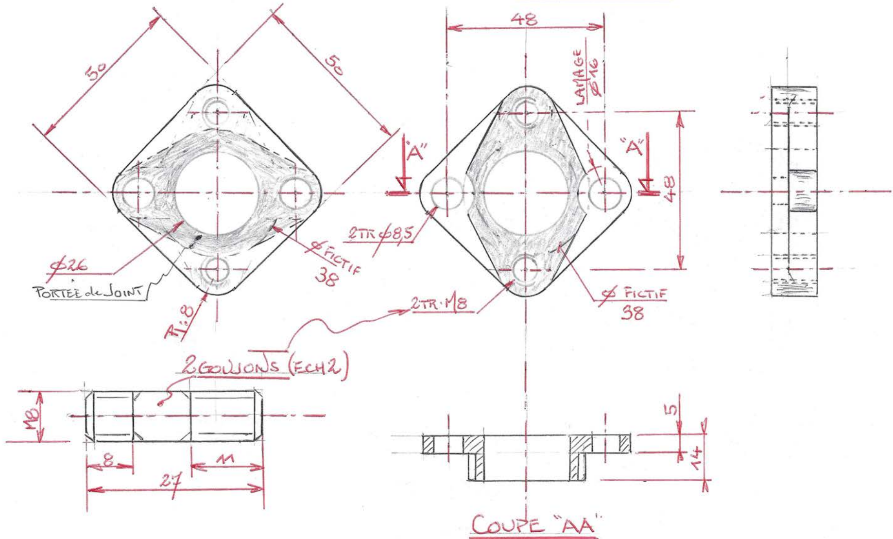
Bride de carburateur Solex \phi 26 - Dessins : Etienne POULALION
